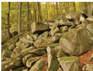
Im Zusammenwirken von geologischen und klimatischen Prozessen über Jahr-millionen hinweg entstand das Felsenmeer. Eckige Blöcke aus Melaspargandit, einem dem Granit sehr ähnlichen Tiefengestein, verwitterten im Untergrund zu gerundeten Blöcken und sammelten sich schließlich in Tälern und Mulden.
