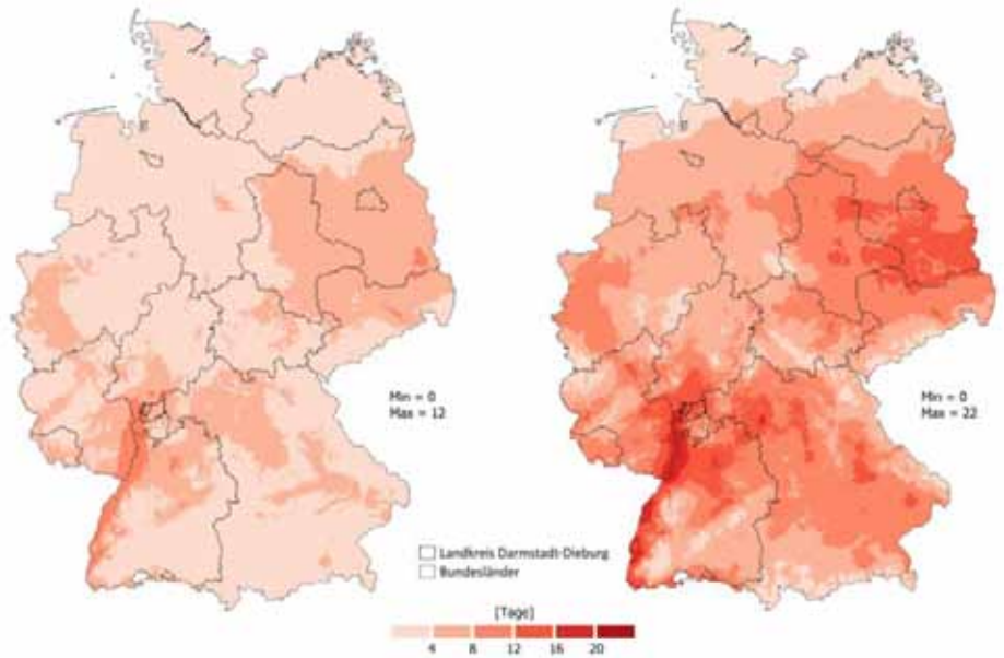
Die Abbildung zeigt den Vergleich der gemittelten Anzahl an Hitzetagen im Referenzzeitraum 1961-1990 links und 1991-2020 rechts. Hitzetage sind Tage an denen die Lufttemperatur mindestens 30 °C beträgt. Quelle: https://www.ladadi.de/umwelt-soziales/natur-bauen/klima/klimaanpassung/ Quelle der Grenzen: © BKG (2026) dl-de/by-2-0, Quelle der Hitzetage: © DWD Climate Data Center (CDC), Jahresraster der Anzahl der Heißen Tage für Deutschland, Version v1.0. (Verändert nach eigenen Berechnungen)
